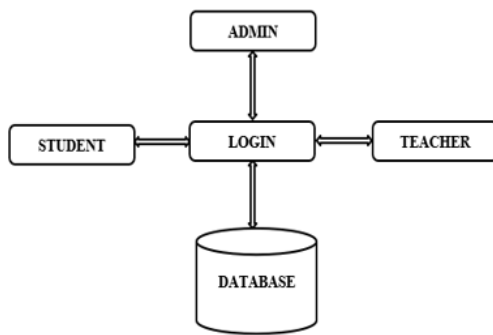
Fig. 2. Users
